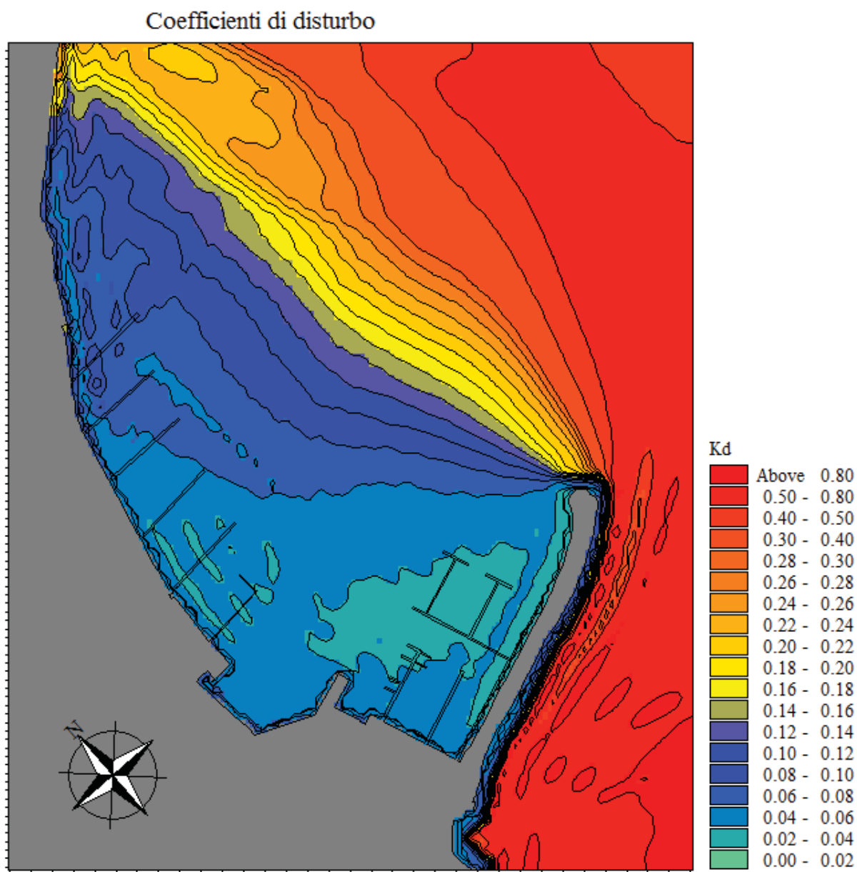
Figura 8 Coefficienti di disturbo T_r = 5 anni stato attuale
