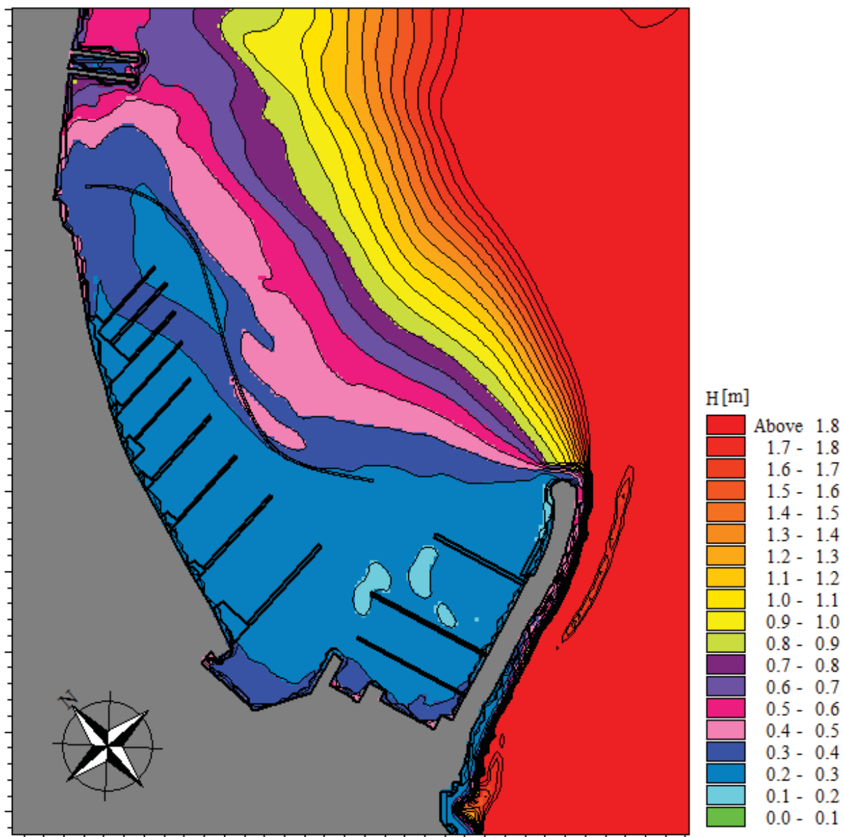
Figura 17 Agitazione ondosa Tr=50anni nuovo progetto
