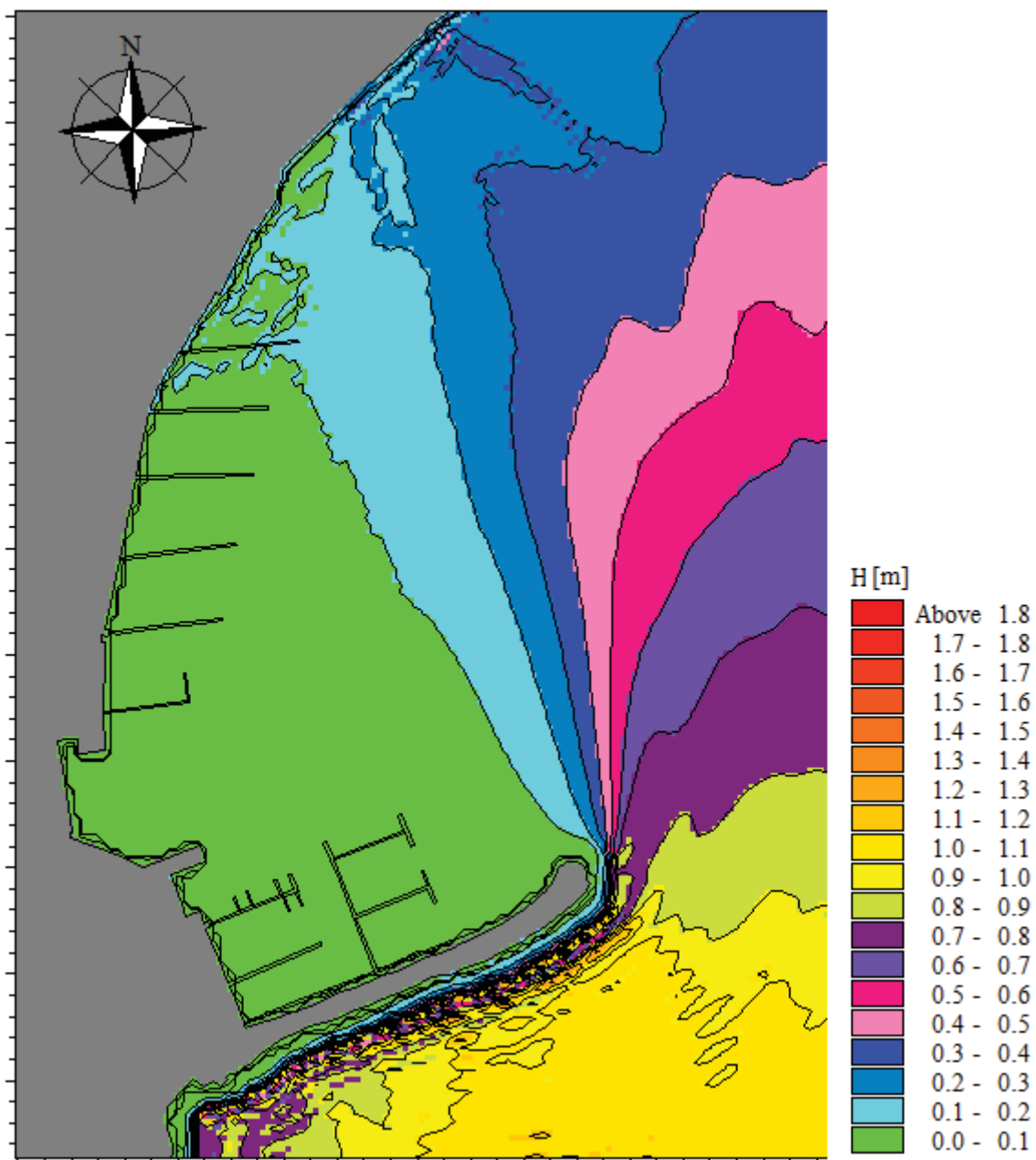
Figura 13 Agitazione ondosa vento 30m/s stato attuale
