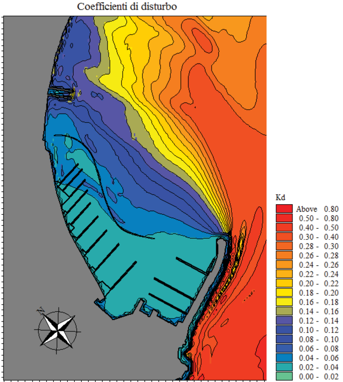
Figura 16 Coefficienti di disturbo T_r = 5 anni nuovo progetto
