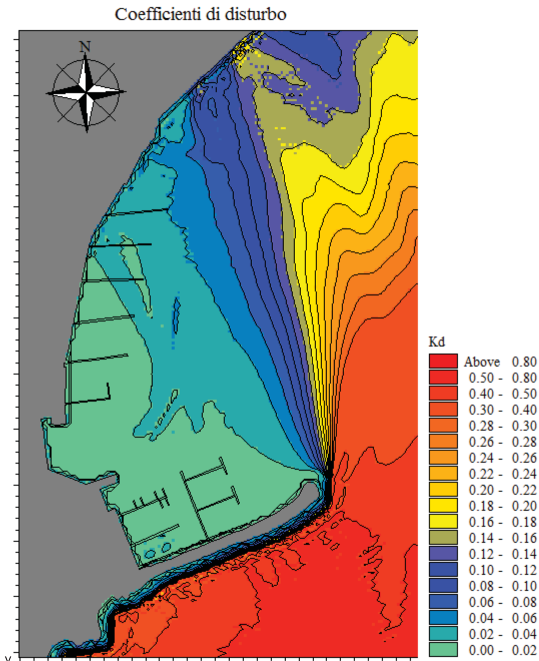
Figura 12 Coefficienti di disturbo vento 20m/s stato attuale
