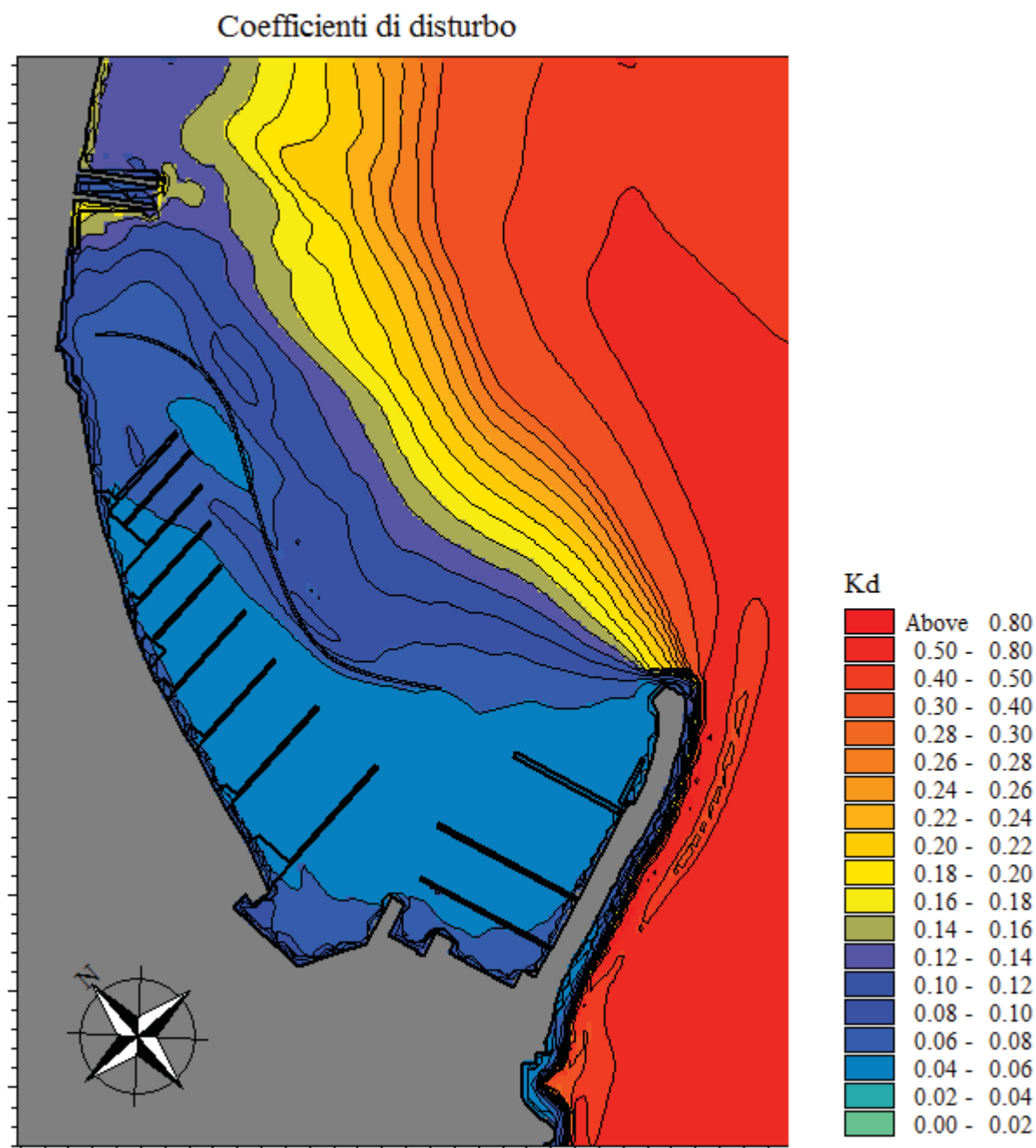
Figura 18 Coefficienti di disturbo T_r=50 anni nuovo progetto
