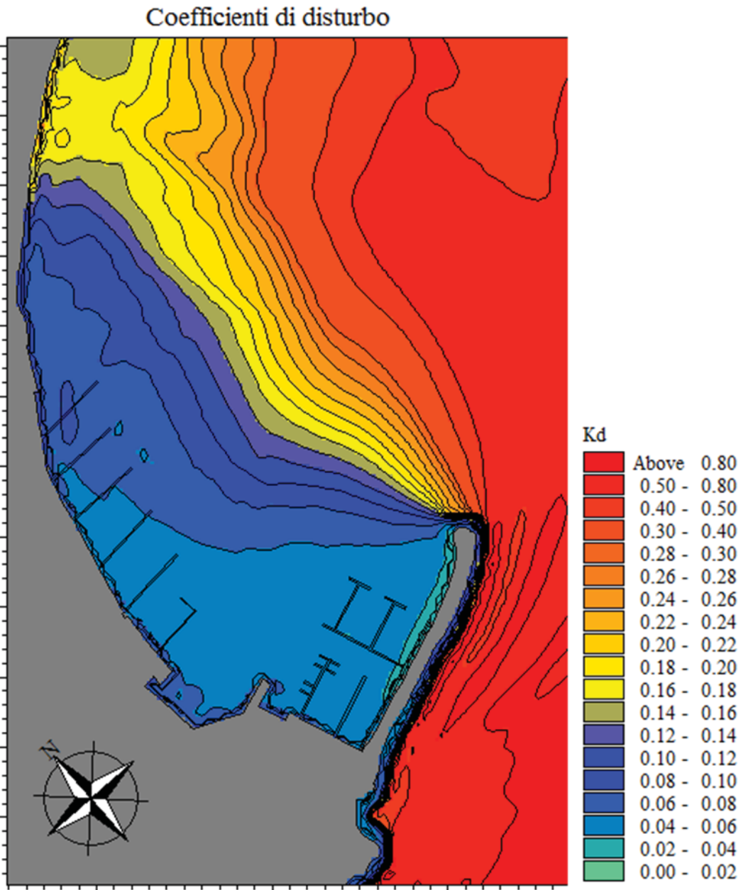
Figura 10 Coefficienti di disturbo T_r = 50 anni stato attuale
