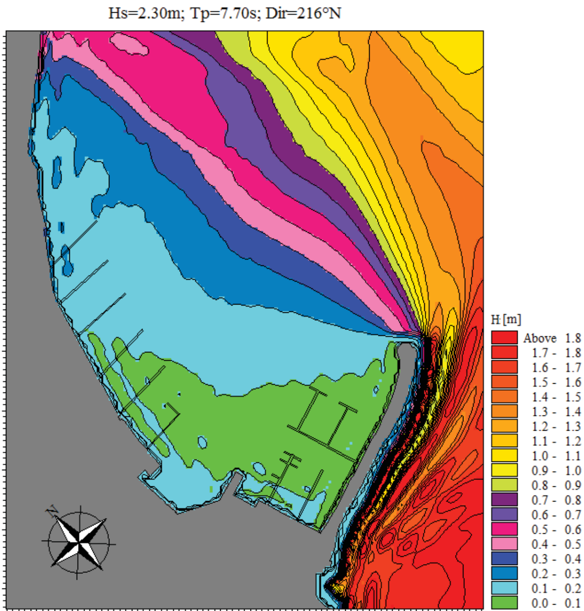
Figura 7 Agitazione ondosa Tr = 5anni stato attuale
