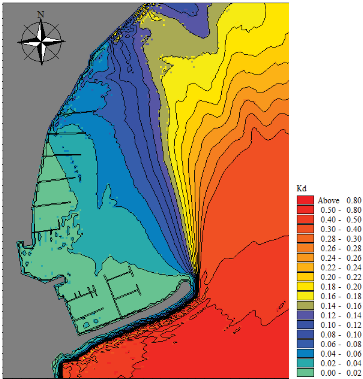
Figura 14 Coefficienti di disturbo vento 30m/s stato attuale
