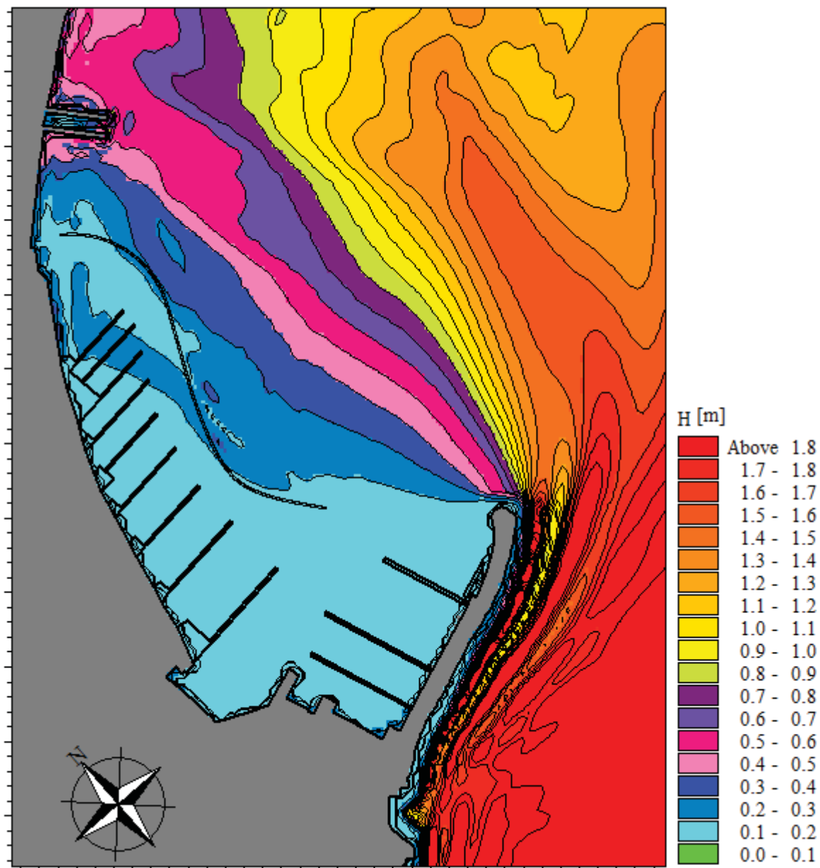
Figura 15 Agitazione ondosa T_r=5 anni nuovo progetto
