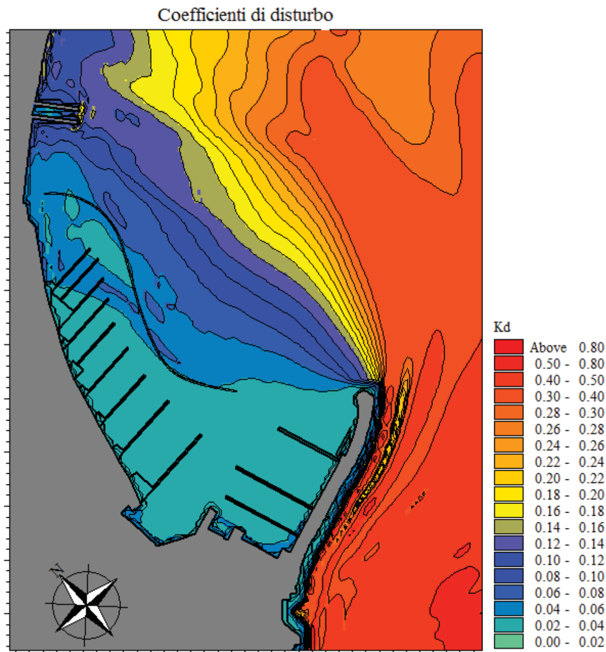
Figura 22 Coefficienti di disturbo vento 30m/s nuovo progetto
