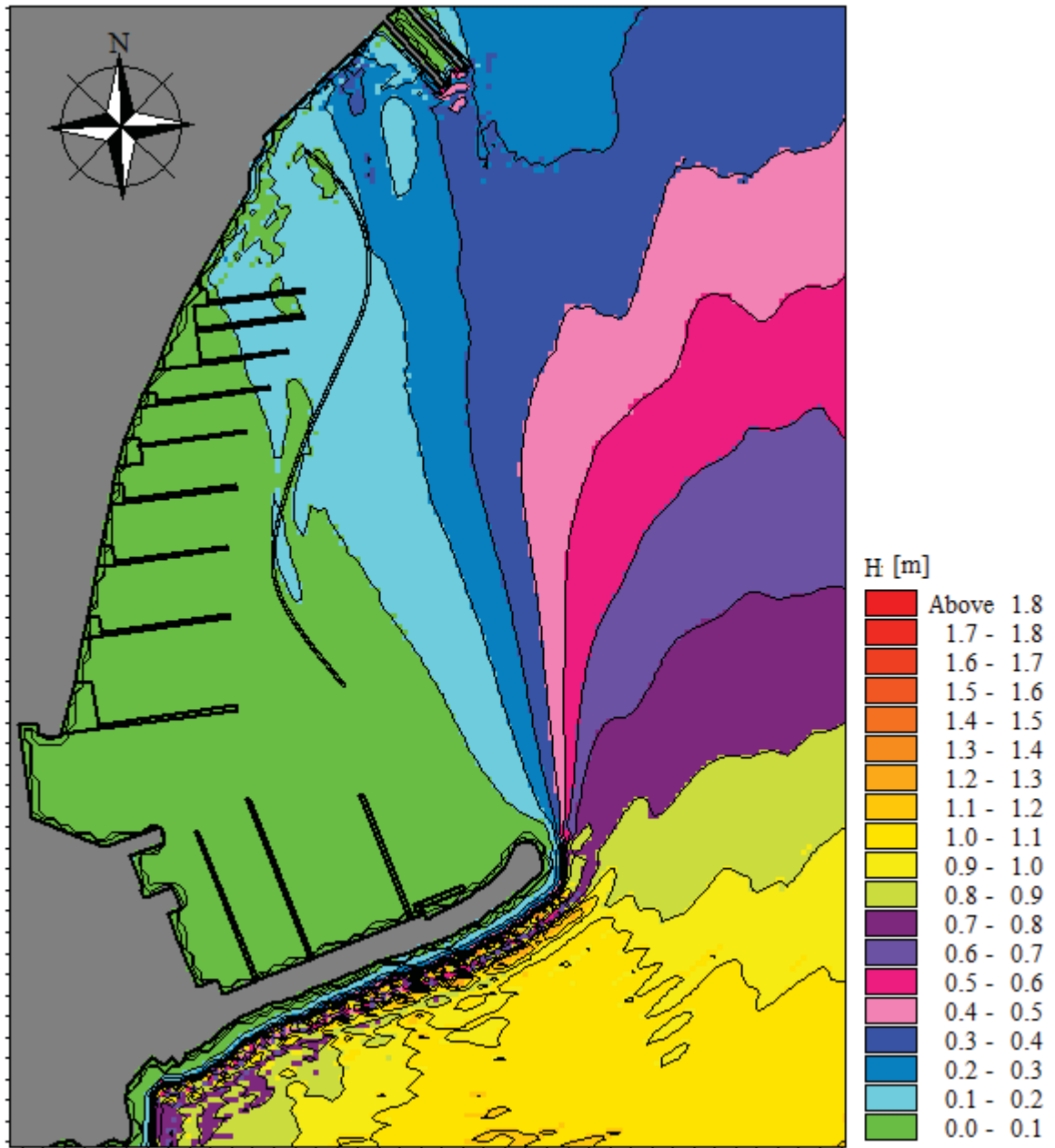
Figura 21 Agitazione ondosa vento 30m/s nuovo progetto
